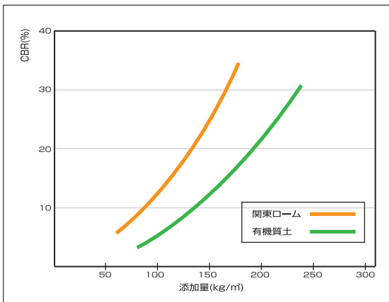
【CBR試験】
